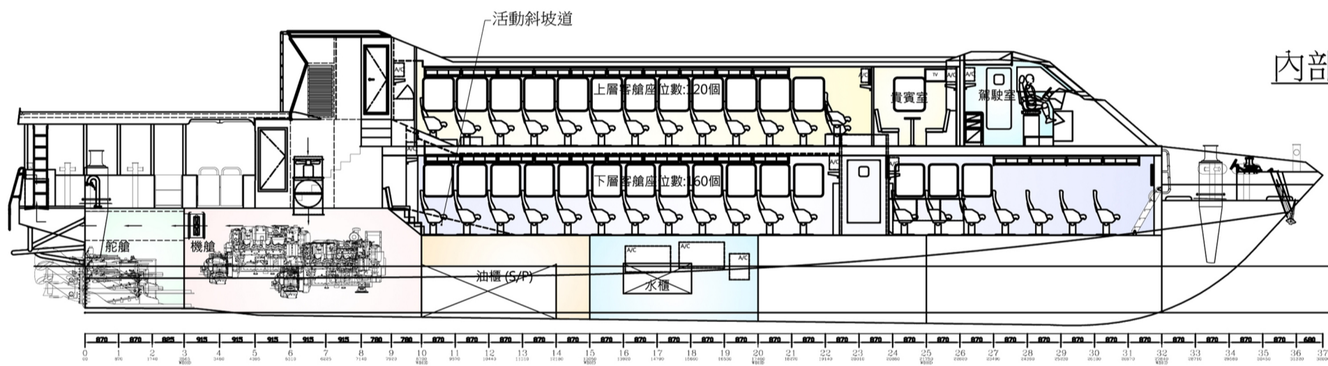
主甲板客艙
